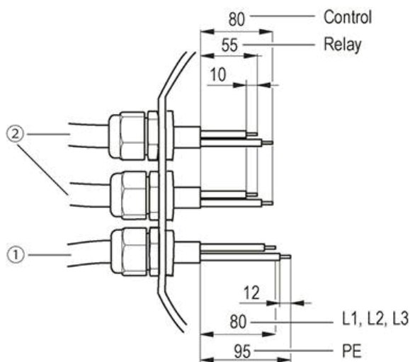
Abb. 1: Empfohlene Abmantellungsgrößen (innerhalb Klemmkasten) (1) Netzleitung (2) Steuer- und Relaisleitung
