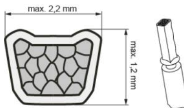
Abb. 2: Trapez-Crimp
