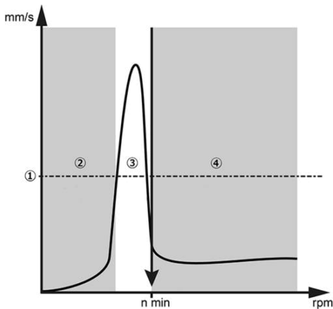
Abb. 7: Schematische Darstellung eines Schwingungsverlaufs
