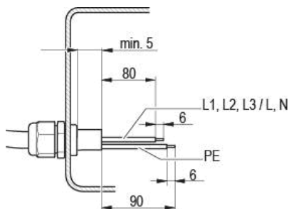
Abb. 2: Empfohlene Abmantelungslängen in mm (innerhalb Klemmkasten)
