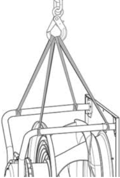
Abb. 1: Hebeskizze für den Transport des RadiPac
