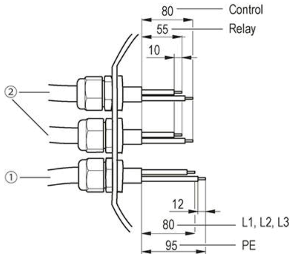
Abb. 1: Empfohlene Abmantellungsgrößen (innerhalb Klemmkasten) (1) Netzleitung (2) Steuer- und Relaisleitung
