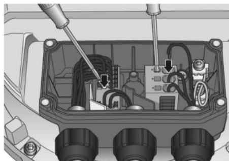
Abb. 4: Anschluss der Leitungen an den Klemmen
