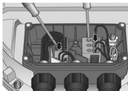
Abb. 5: Anschluss der Leitungen an den Klemmen
