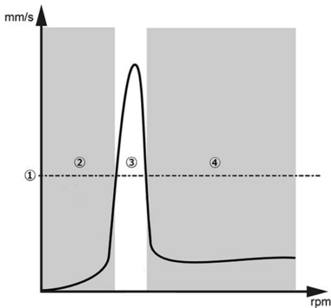
Abb. 7: Schematische Darstellung eines Schwingungsverlaufs Überprüfung des Ventilators auf mechanische Schwingungen in Anlehnung an die ISO 14694. Empfehlung: Alle 6 Monate. Hinweise siehe Kapitel 4.10 Ausblenden von Drehzahlbereichen. (1) Grenzwert, darüber ist eine Schädigung der Lager zu erwarten. (2) Bereich unterhalb der Resonanzfrequenz: Im Bereich unter der Resonanzfrequenz liegt die Schwingstärke unterhalb des zulässigen Grenzwertes. (3) Bereich in der Nähe der Resonanzfrequenz: In diesem Drehzahlbereich liegt die Schwinggeschwindigkeit teilweise deutlich über dem zulässigen Grenzwert. Ein längerer Betrieb in diesem Bereich reduziert die Gesamtlebensdauer. Dieser Drehzahlbereich ist so schnell wie möglich zu durchfahren und ein dauerhafter Betrieb sollte unbedingt vermieden werden. (4) Bereich oberhalb der Resonanzfrequenz: In ausreichendem Abstand zur Resonanzspitze liegt der ideale Drehzahlbereich des Ventilators, in dem der Schwingungspegel deutlich unterhalb des Grenzwertes liegt.
