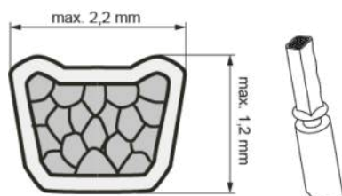
Abb. 3: Trapez-Crimp
