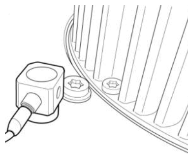
Abb. 6: ebm-papst empfiehlt die Verwendung eines Schwingungssensors, der von einem Messpunkt ausgehend in alle drei Richtungen misst (triaxialer Messaufnehmer).
