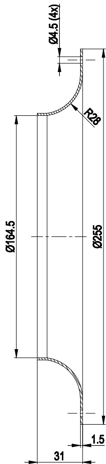
Einströmdüse 96359-2-4013
