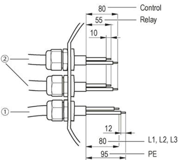
Abb. 2: Empfohlene Abmantelungslängen (innerhalb Klemmkasten) (1) Netzleitung (2) Steuer- und Relaisleitung
