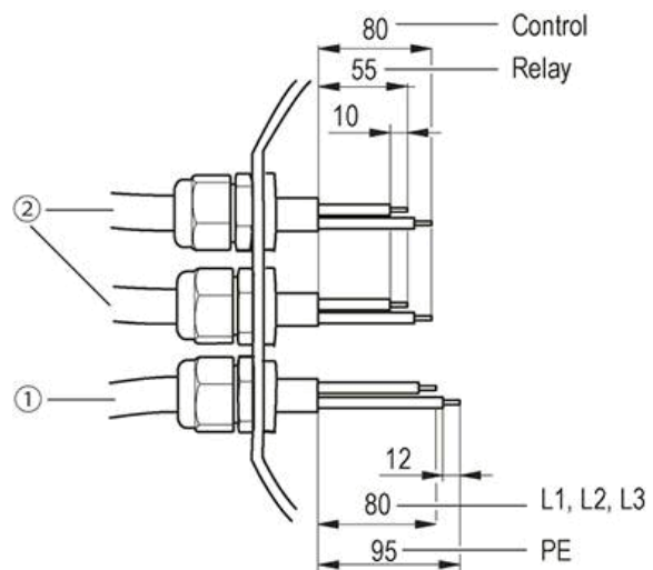
Abb. 2: Empfohlene Abmantellungs- (innerhalb Klemmkasten) (1) Netzleitung (2) Steuer- und Relaisleitung
