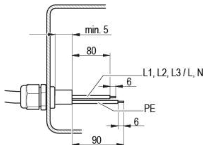
Abb. 1: Empfohlene Abmangelungslängen in mm (innerhalb Klemmkasten)
