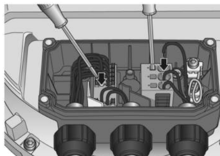
Abb. 3: Anschluss der Leitungen an den Klemmen
