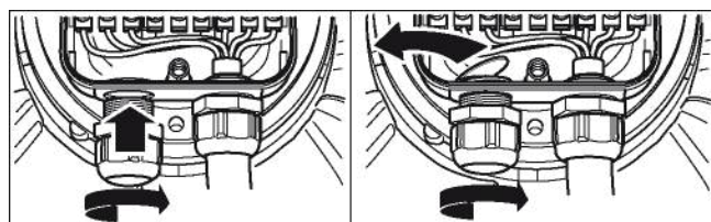
Abb. 4: Durchbruch Kabelverschraubung
