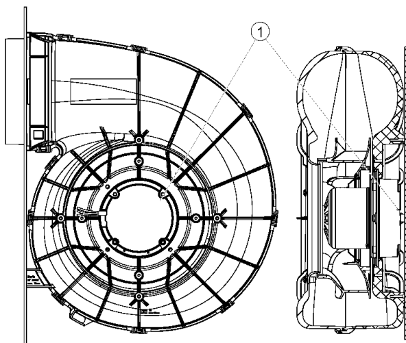
Abb. 1: Ventilator im eingebauten Zustand
