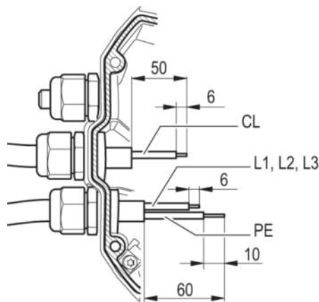
Abb. 2: Empfohlene Abmantellungsabstände in mm (innerhalb Klemmkasten)
