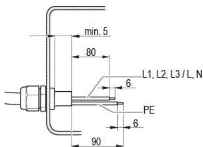
Abb. 2: Empfohlene Abmantellungsgrößen in mm (innerhalb Klemmkasten)
