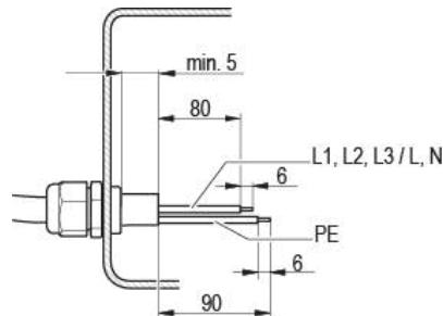
Abb. 2: Empfohlene Abmangelungslängen in mm (innerhalb Klemmkasten)
