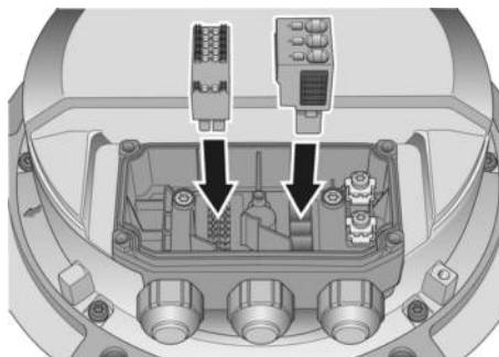
Abb. 3: Montieren Sie die Steckverbinder im Klemmkasten
