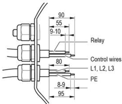
Abb. 2: Empfohlene Abmantelungslängen in mm (innerhalb Klemmkasten)
