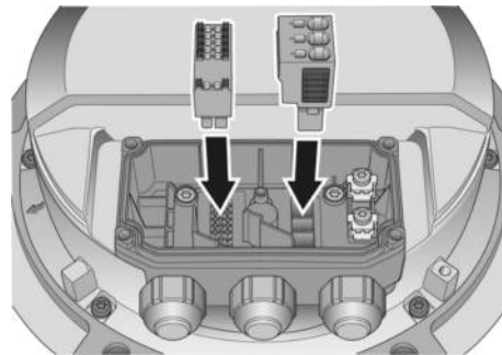
Abb. 3: Montieren Sie die Steckverbinder im Klemmkasten
