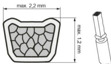
Abb. 3: Trapez-Crimp
