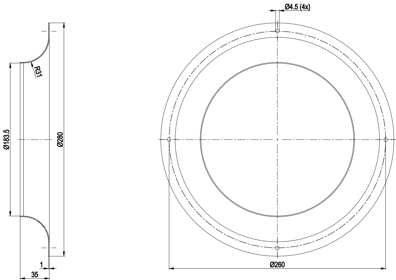
Einströmdüse 96360-2-4013
