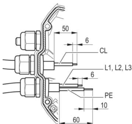
Abb. 1: Empfohlene Abmantellungsängen in mm (innerhalb Klemmkasten)
