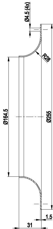
Einströmdüse 96359-2-4013
