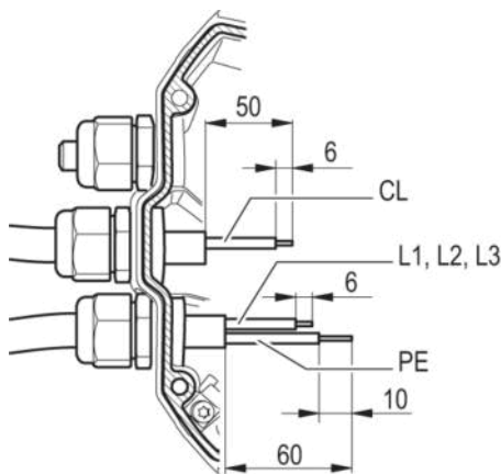
Abb. 1: Empfohlene Abmantellungsängen in mm (innerhalb Klemmkasten)
