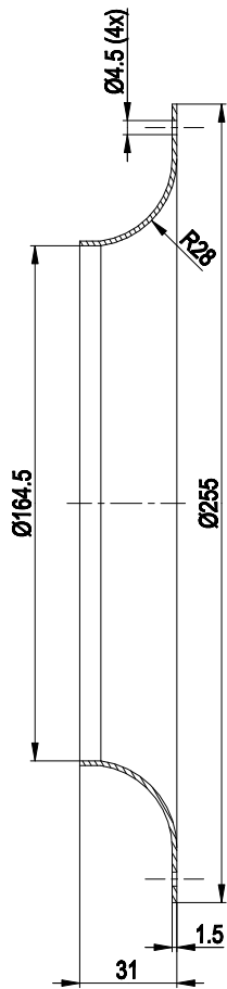
Einströmdüse 96359-2-4013
