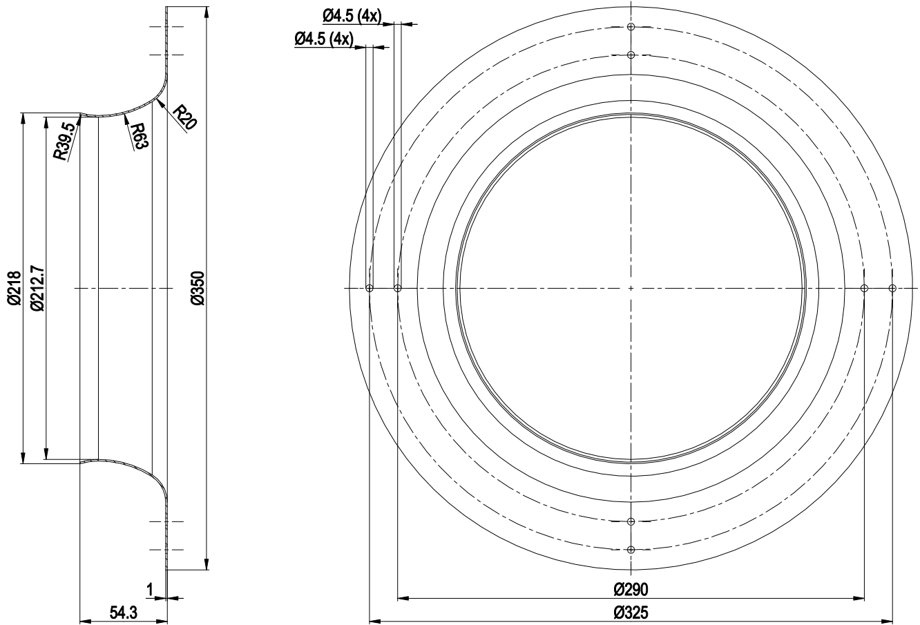
Einströmdüse 31570-2-4013
