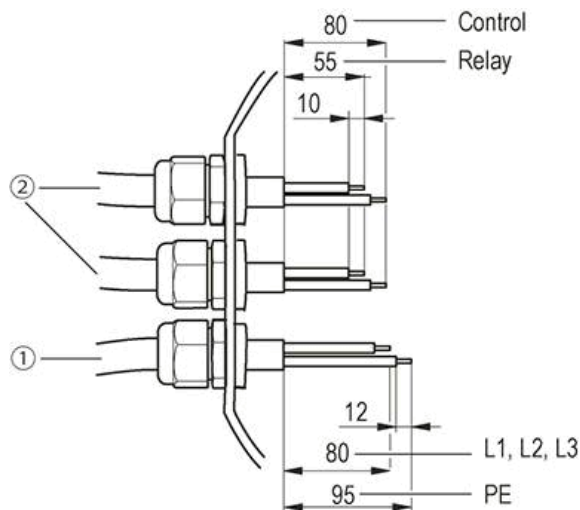
Abb. 1: Empfohlene Abmantellungsängen (innerhalb Klemmkasten) (1) Netzleitung (2) Steuer- und Relaisleitung
