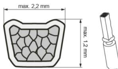
Abb. 2: Trapez-Crimp
