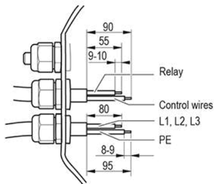
Abb. 1: Empfohlene Abmantelllängen in mm (innerhalb Klemmkasten)
