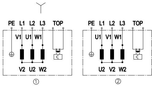
Drehrichtungsänderung durch Vertauschen von zwei Phasen
