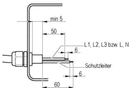
Abb. 1: Empfohlene Abmantellungslängen in mm (innerhalb Klemmkasten)
