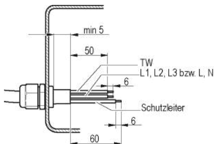
Abb. 1: Empfohlene Abmantellungsanordnungen in mm (innerhalb Klemmkasten)
