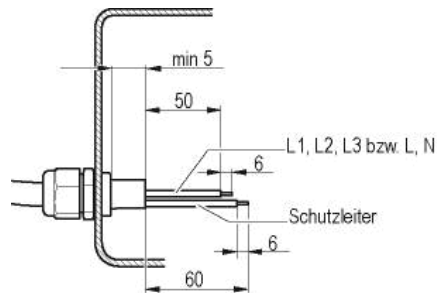
Abb. 1: Empfohlene Abmantellungsabstände in mm (innerhalb Klemmkasten)
