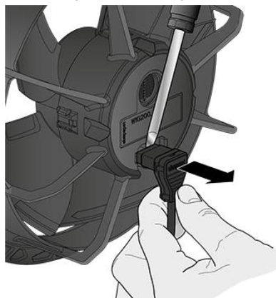
Abb. 3: Verwenden Sie zum Lösen der Steckverbindung einen Schraubendreher. Mit diesem kann der Stecker gerade herausgehoben werden.
