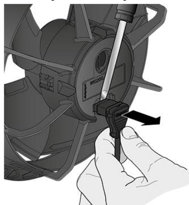
Abb. 3: Verwenden Sie zum Lösen der Steckverbindung einen Schraubendreher. Mit diesem kann der Stecker gerade herausgehoben werden.
