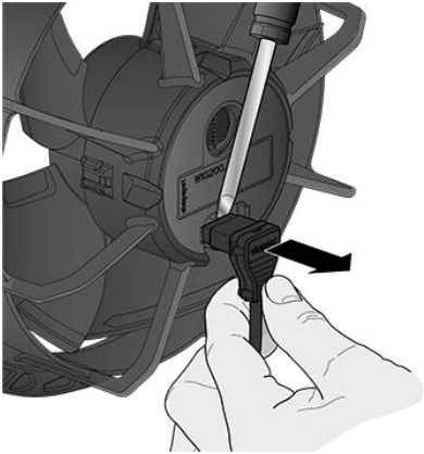
Abb. 5: Verwenden Sie zum Lösen der Steckverbindung einen Schraubendreher. Mit diesem kann der Stecker gerade herausgeholt werden. Vorsicht! Schräges Herausziehen kann die Anschlüsse am Ventilator beschädigen!
