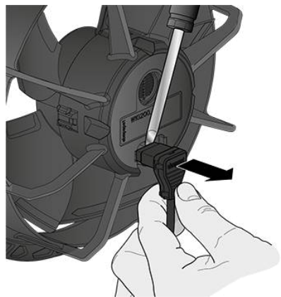
Abb. 2: Verwenden Sie zum Lösen der Steckverbindung einen Schraubendreher. Mit diesem kann der Stecker gerade herausgehoben werden.
