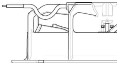
Abb. 3: Liegend eingebauter Ventilator, Verlegung des Kabels als Wassersack.
