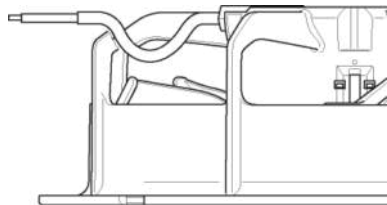
Abb. 1: Liegend eingebauter Ventilator, Verlegung des Kabels als Wassersack.
