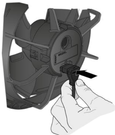
Abb. 4: Beim Einstecken des Steckers darauf achten, dass dieser gerade eingeführt wird. Ein schräg angesetzter Stecker kann zu Beschädigungen an der Verbindung am Ventilator führen.
