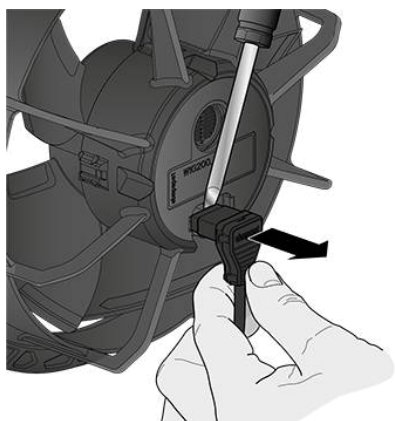
Abb. 3: Verwenden Sie zum Lösen der Steckverbindung einen Schraubendreher. Mit diesem kann der Stecker gerade herausgehebelt werden.
