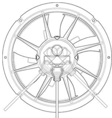
Abb. 2: Kabelverlegung bei stehend eingebauten Ventilatoren.
