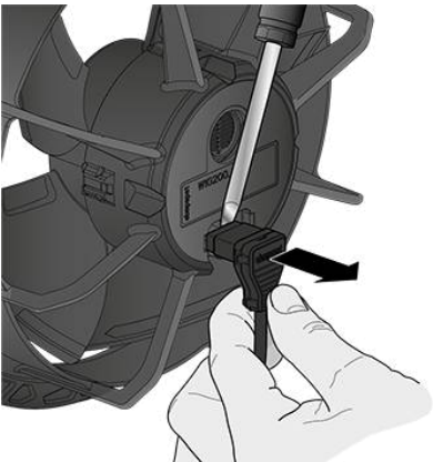
Abb. 3: Verwenden Sie zum Lösen der Steckverbindung einen Schraubendreher. Mit diesem kann der Stecker gerade herausgehebelt werden. Vorsicht! Schräges Herausziehen kann die Anschlüsse am Ventilator beschädigen!
