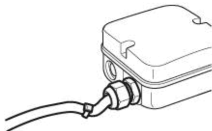
Abb. 1: Liegend eingebauter Ventilator, Verlegung des Kabels als Wassersack (beispielhafte Darstellung).
