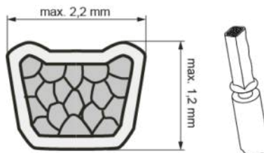
Abb. 2: Trapez-Crimp
