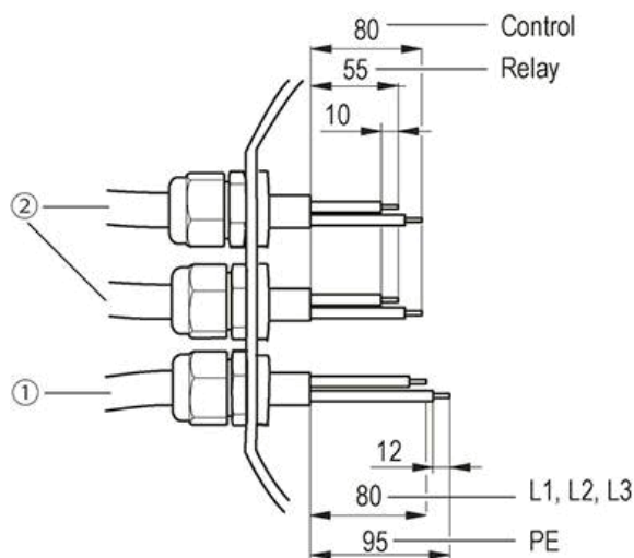
Abb. 1: Empfohlene Abmantelungslängen (innerhalb Klemmkasten) (1) Netzleitung (2) Steuer- und Relaisleitung
