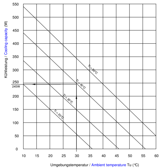
Leistungsdiagramm / Performance curve PK 150
