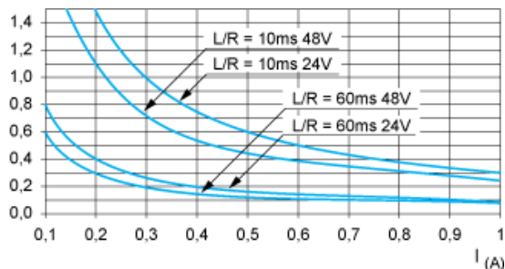
DC13-Kurven
