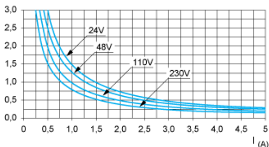
AC12-Kurven
