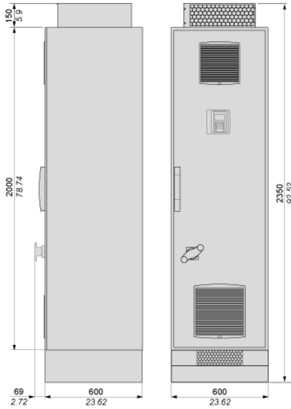
Rechtsseitige Ansicht und Vorderansicht
