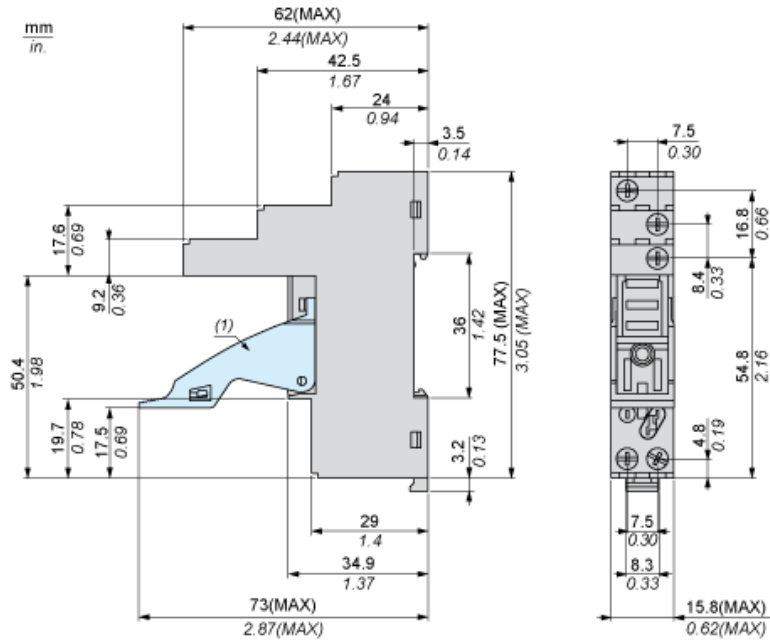
(1) Befestigungsklammer
