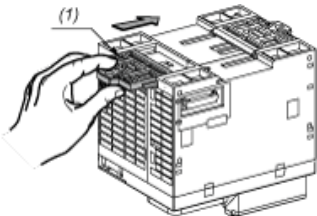
(1) Montieren eines Montagebandes
