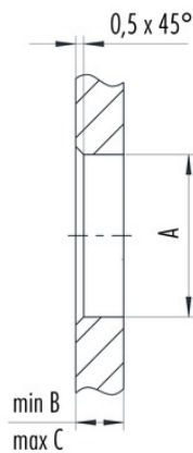
Mit Durchgangsbohrung
