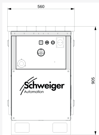
Frontansicht
