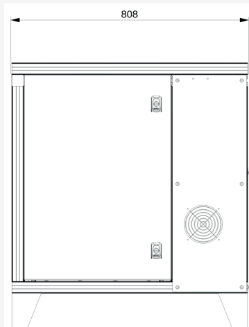
Seitliche Ansicht
